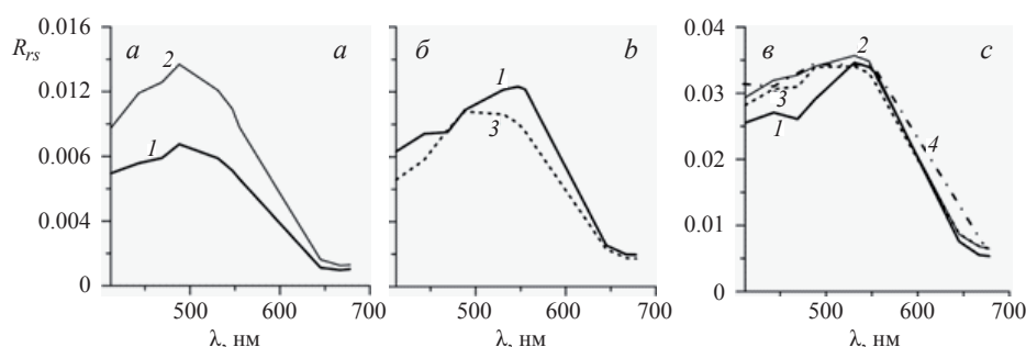
Рис. 3. Сопоставление данных спутниковых измерений спектрального коэффициента яркости моря R_{rs}(\lambda) с данными судовых измерений плавающим спектрорадиометром (кривые 1) на трех станциях в Баренцевом море: ст. 5576 (а), ст. 5577 (б) и ст. 5580 (в). Кривые 2 — данные сканера MODIS-Aqua, 3 — MODIS-Terra, 4 — VIIRS.
