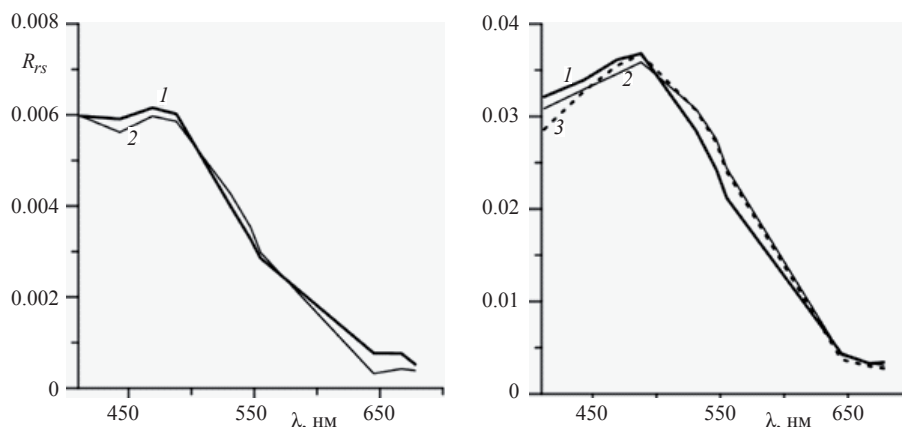
Рис. 2. Сопоставление данных спутниковых измерений спектрального коэффициента яркости моря R_{rs}(\lambda) с данными судовых измерений палубным спектрометриком на двух станциях в Баренцевом море: ст. 6527 (а) вне зоны цветения, ст. 6531 (б) — в зоне. Кривые 1 — измерения палубным спектрометриком, кривые 2 — данные сканера MODIS-Aqua, кривые 3 — MODIS-Terra.
