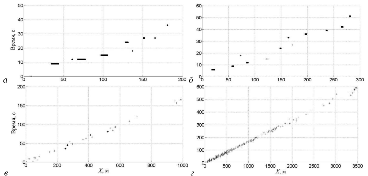
Рис. 10. Срез волнового поля на уровне троекратного превышения значительной амплитуды. Объяснение a–г – см.рис. 3. Для удобства выбран разный масштаб.
