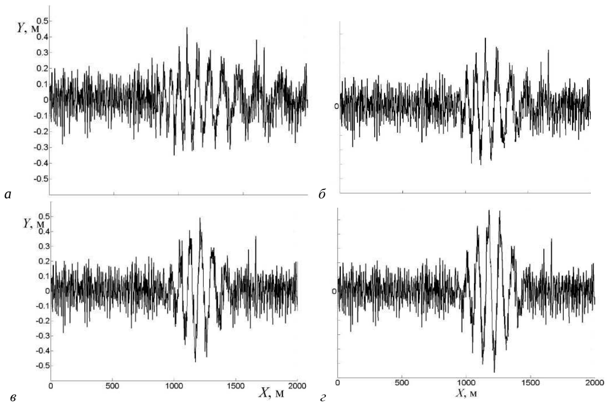
Рис. 8. Наложение волн зыби и ветровых волн в момент времени 200 с для различной формы anomalной волны зыби. Объяснение а-г – см.рис. 3.
