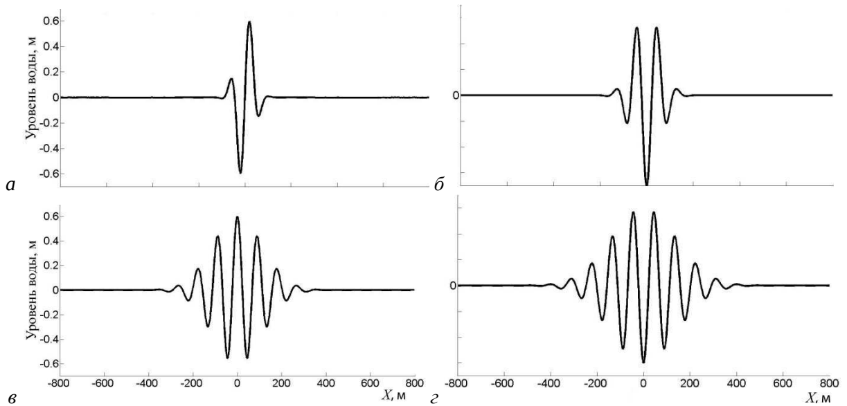
Рис. 2. Начальные возмущения разных форм в нулевой момент времени. а – «одна сестра» ( a = 0.72 м, l = 50 м); б – группа аномальных волн типа «две сестры» ( a = 0.8 м, l = 80 м); в – «три сестры» ( a = 0.59 м, l = 160 м); г – «четыре сестры» ( a = -0.62 м, l = 200 м).
