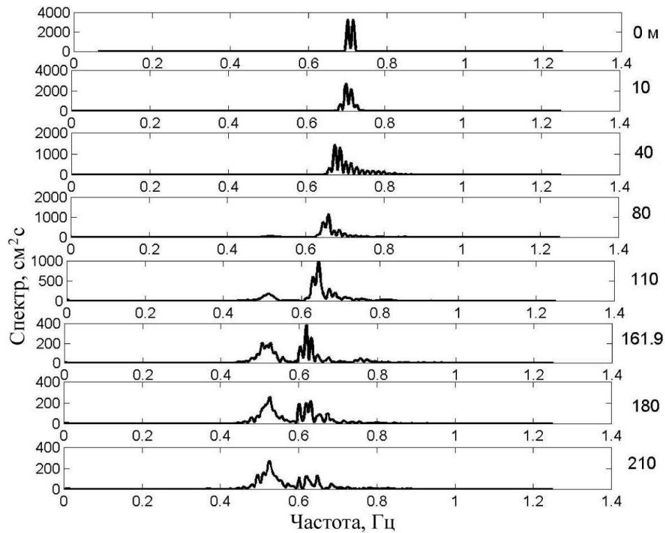
Рис. 5. Пространственная эволюция спектра волнения (рис. 1).
