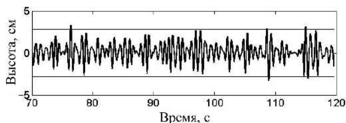
Рис. 3. Хронограмма изначально монохроматической волны с начальной амплитудой 4 см и частотой 1.55 Гц на 38 м после начала ее трансформации. Горизонтальные линии определяют область, соответствующую 2H_{sig} .
